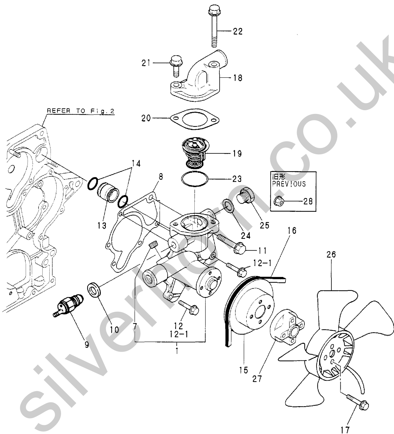
Fig. 9 冷却水システム COOLING WATER SYSTEM
