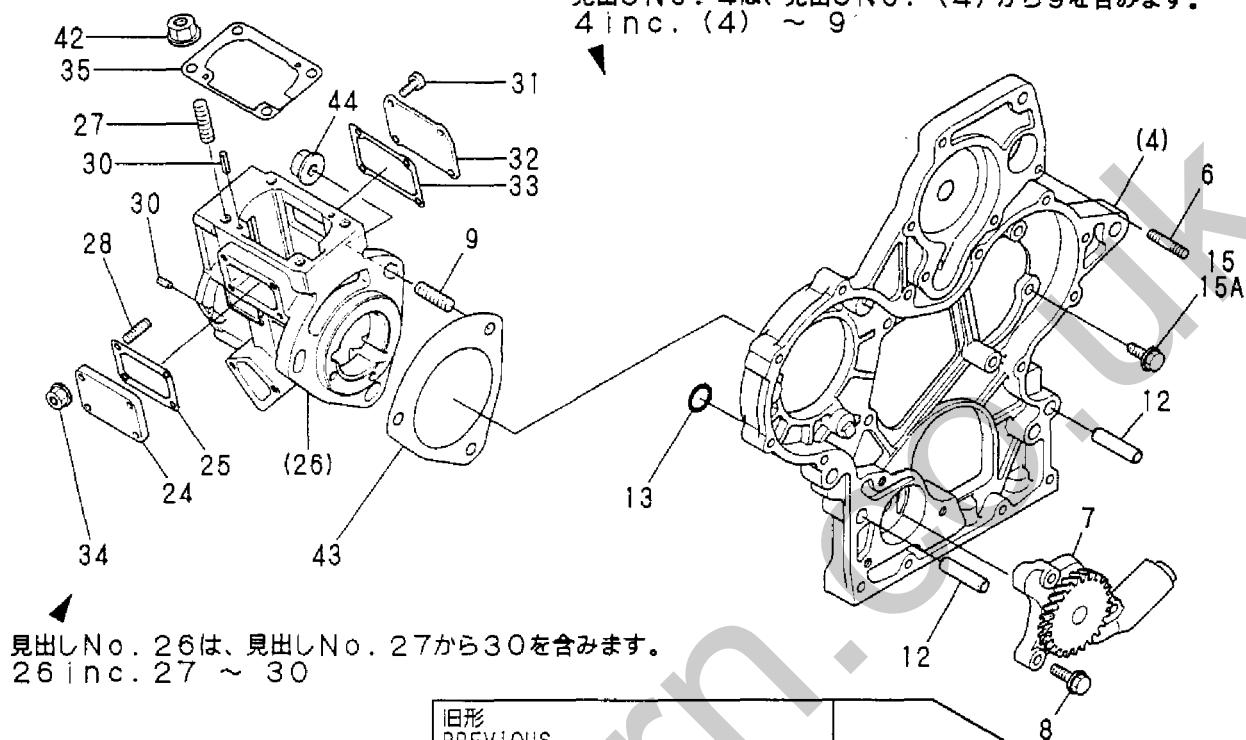
Fig. 2 ギヤケース GEAR HOUSING
