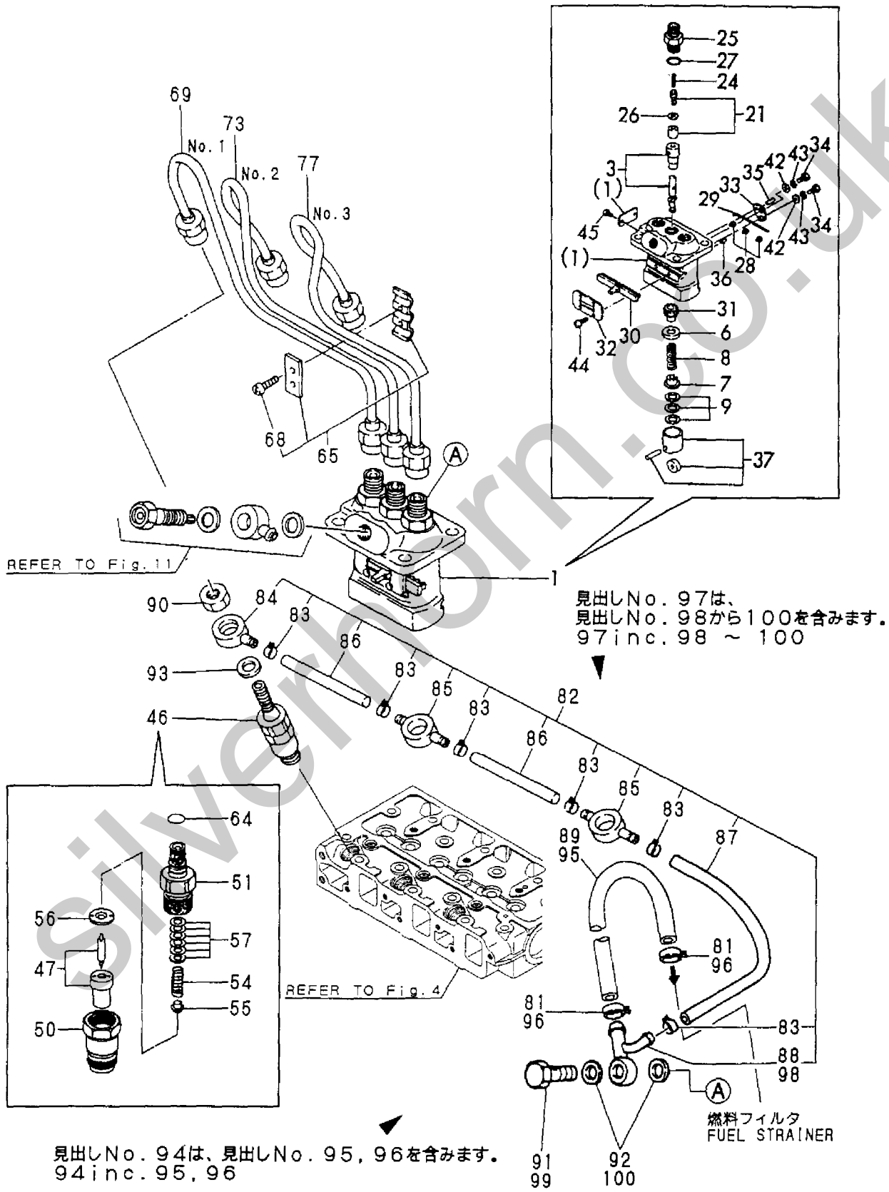
Fig. 10 燃料噴射装置 FUEL INJECTION DEVICE
