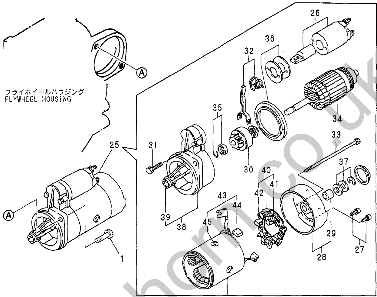
Fig. 13 スターティングモータ STARTING MOTOR
