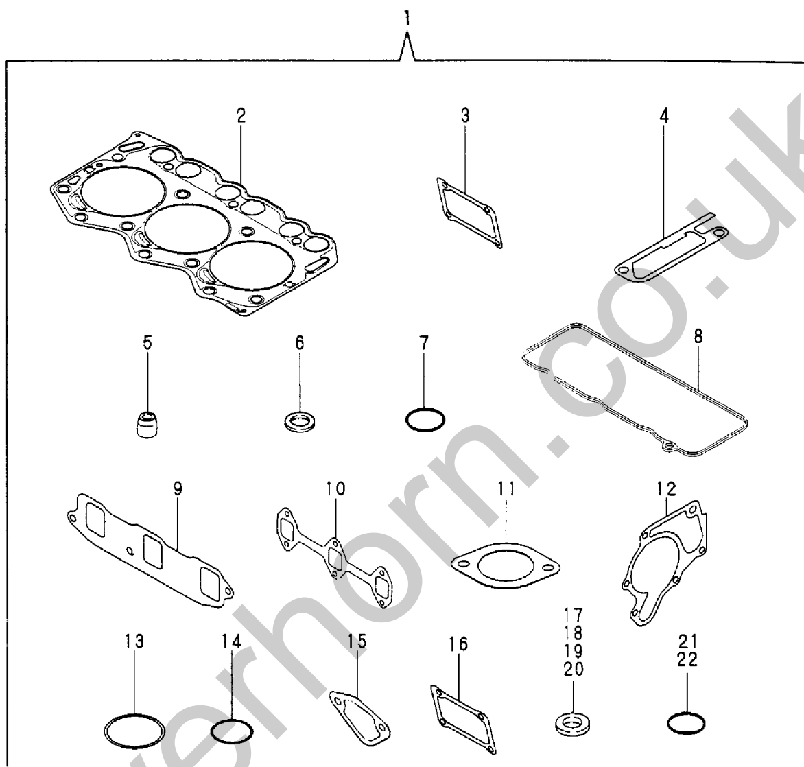
Fig. 15 パッキンセット (オプション) & 工具 GASKET SET (OPTIONAL) & TOOL
