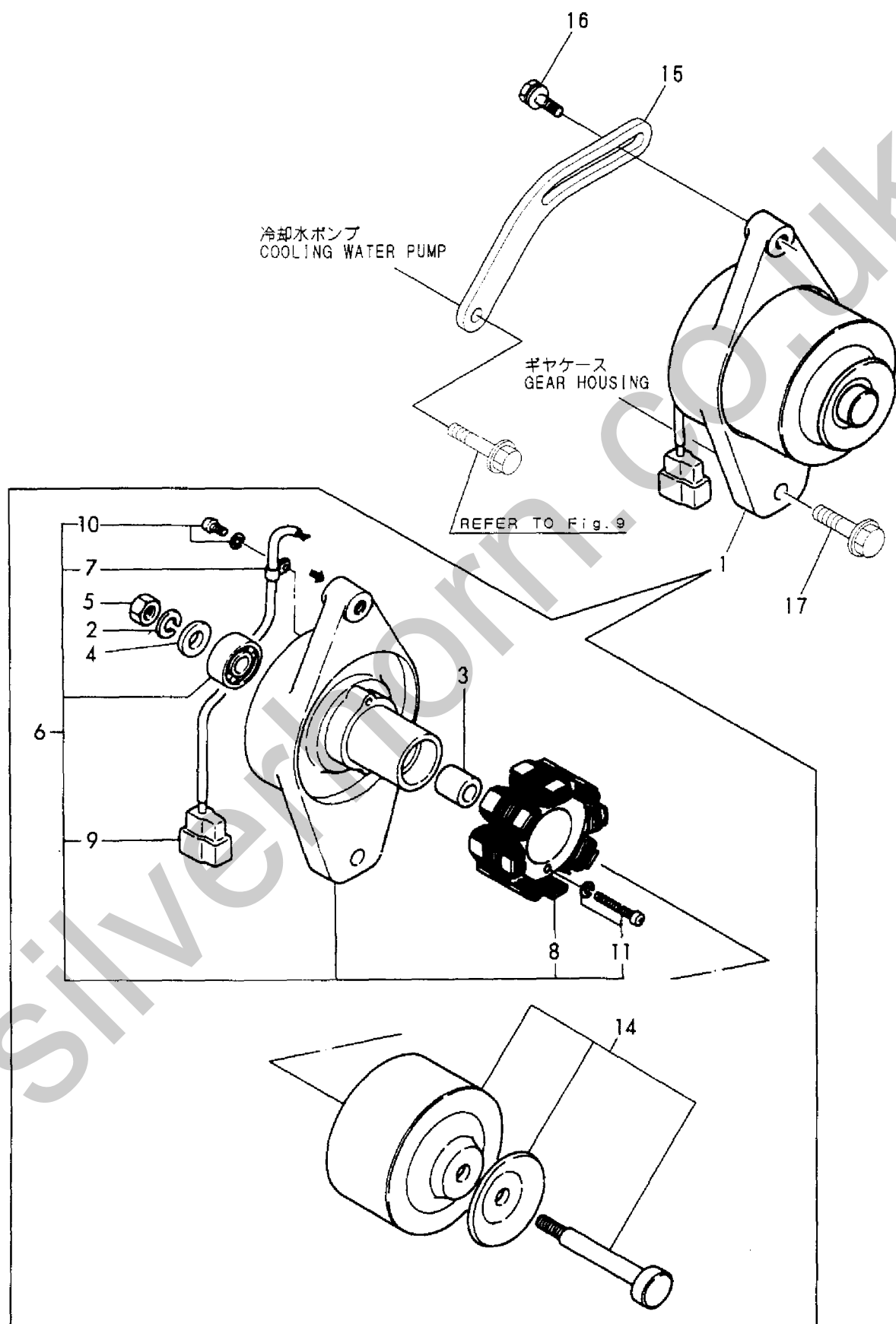
Fig. 14 ジェネレータ GENERATOR
